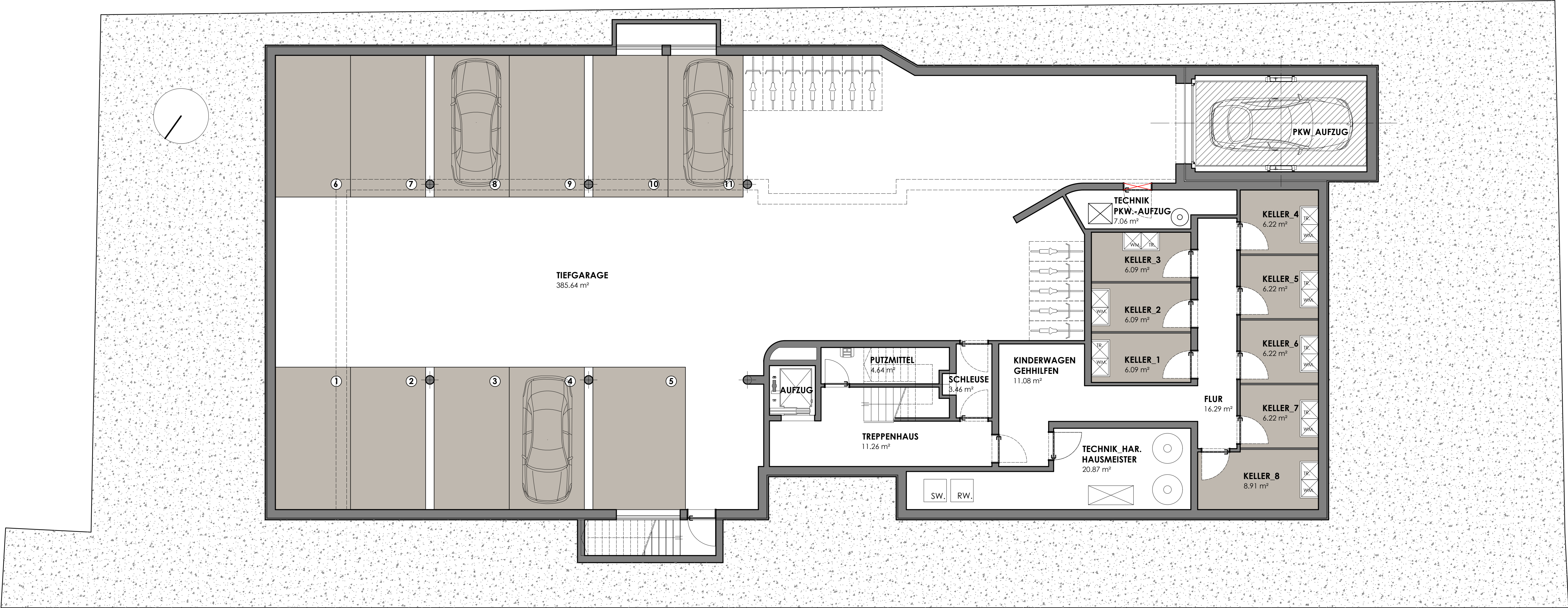
GRUNDRISS_UNTERGESCHOSS
